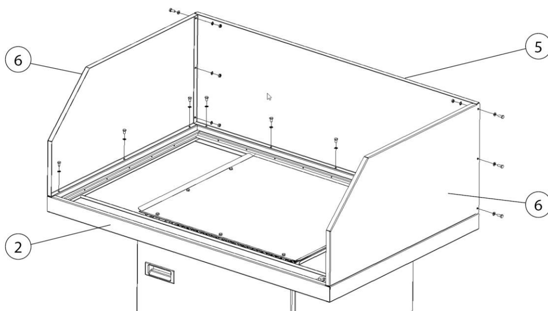
Fig. 4 : montage des parois latérales + panneau arrière
