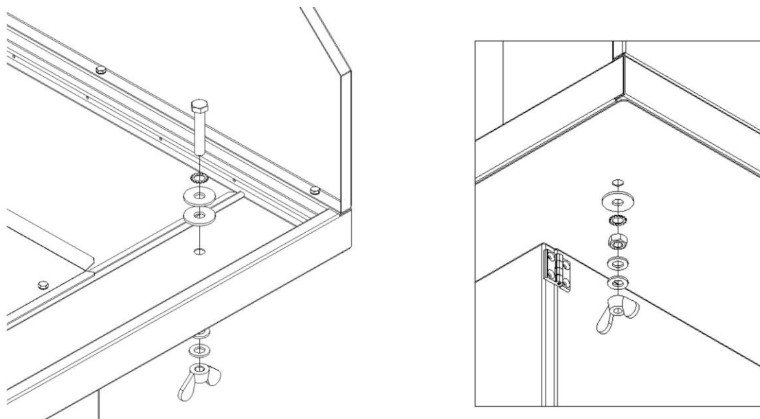
Fig. 5 : montage de la vis de mise à la terre
