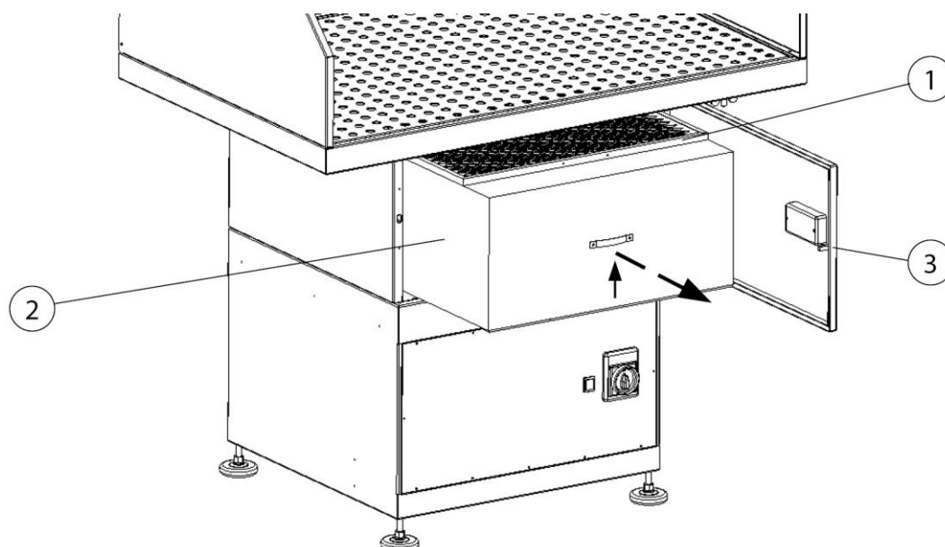
Fig. 10 : remplacement du filtre – Préfiltre + Filtre principal
