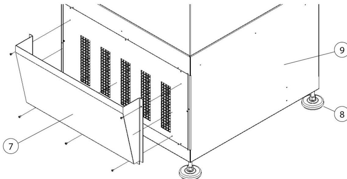
Fig. 6 : montage de la caisse de sortie d'air
