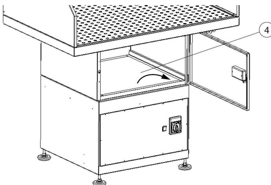
Fig. 11 : remplacement du filtre – Filtre à charbon actif (en option)
