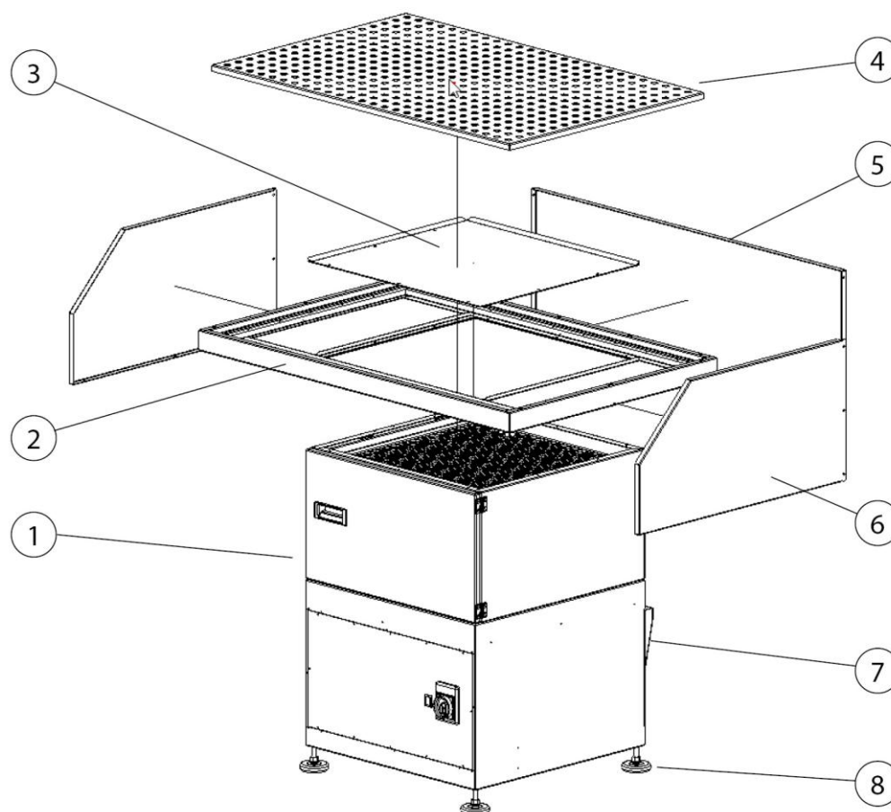
Fig. 2 : montage
