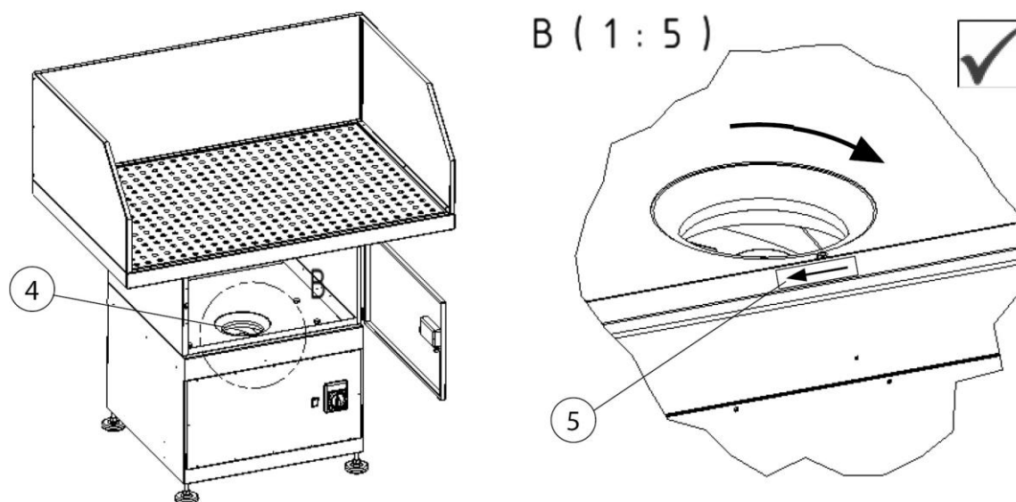
Fig. 8 : contrôle du sens de rotation de la roue à ailettes du ventilateur
