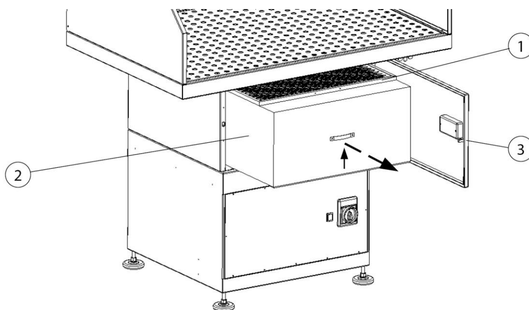
Fig. 7 : contrôle du sens de rotation du ventilateur
